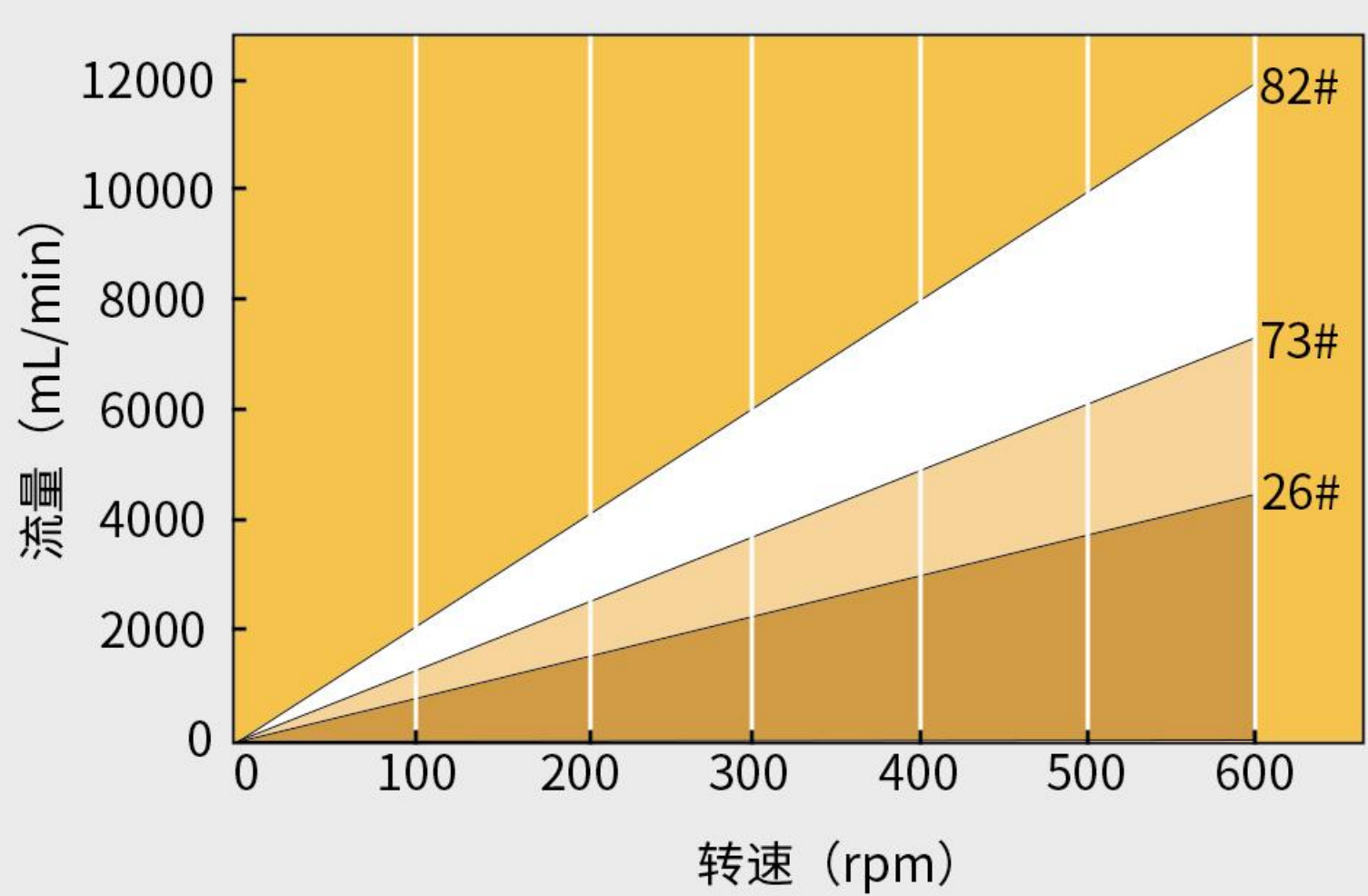
YZ35-II泵头流量范围 (0.1-600rpm)
