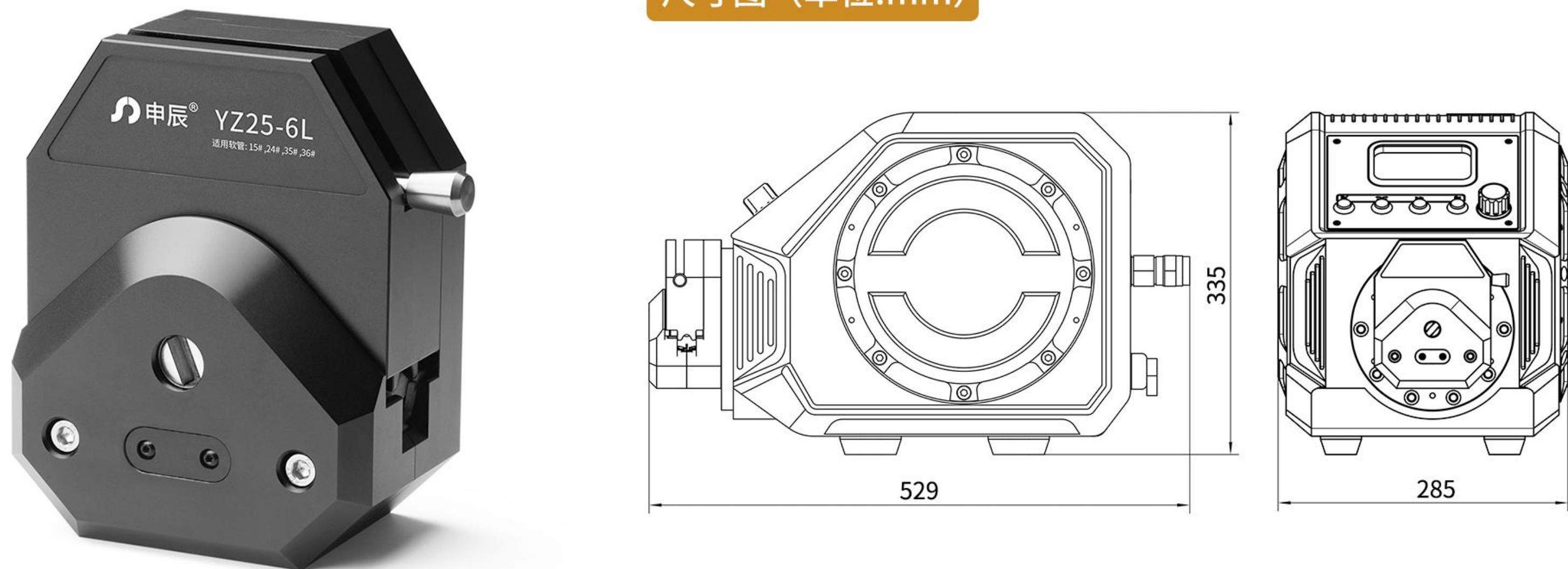
尺寸图 (单位:mm)
