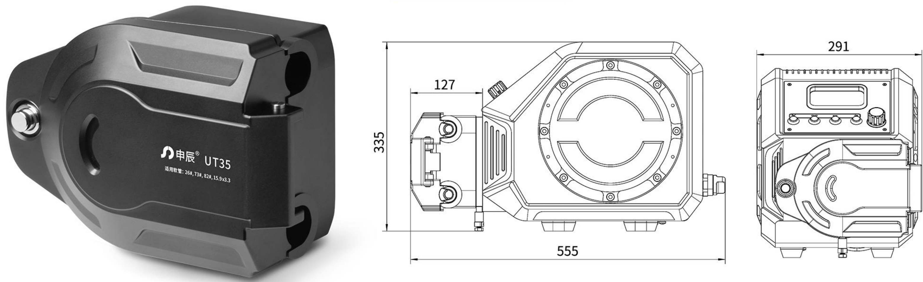
尺寸图 (单位:mm)
