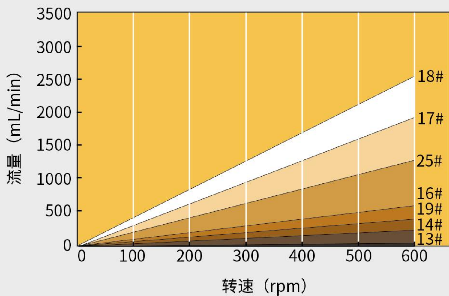
DZ15-3L泵头灌装精度表
