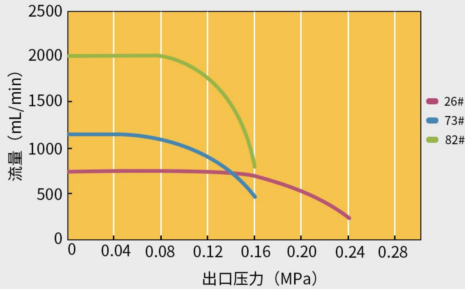
YZ35-II泵头压力曲线图 (100rpm)
