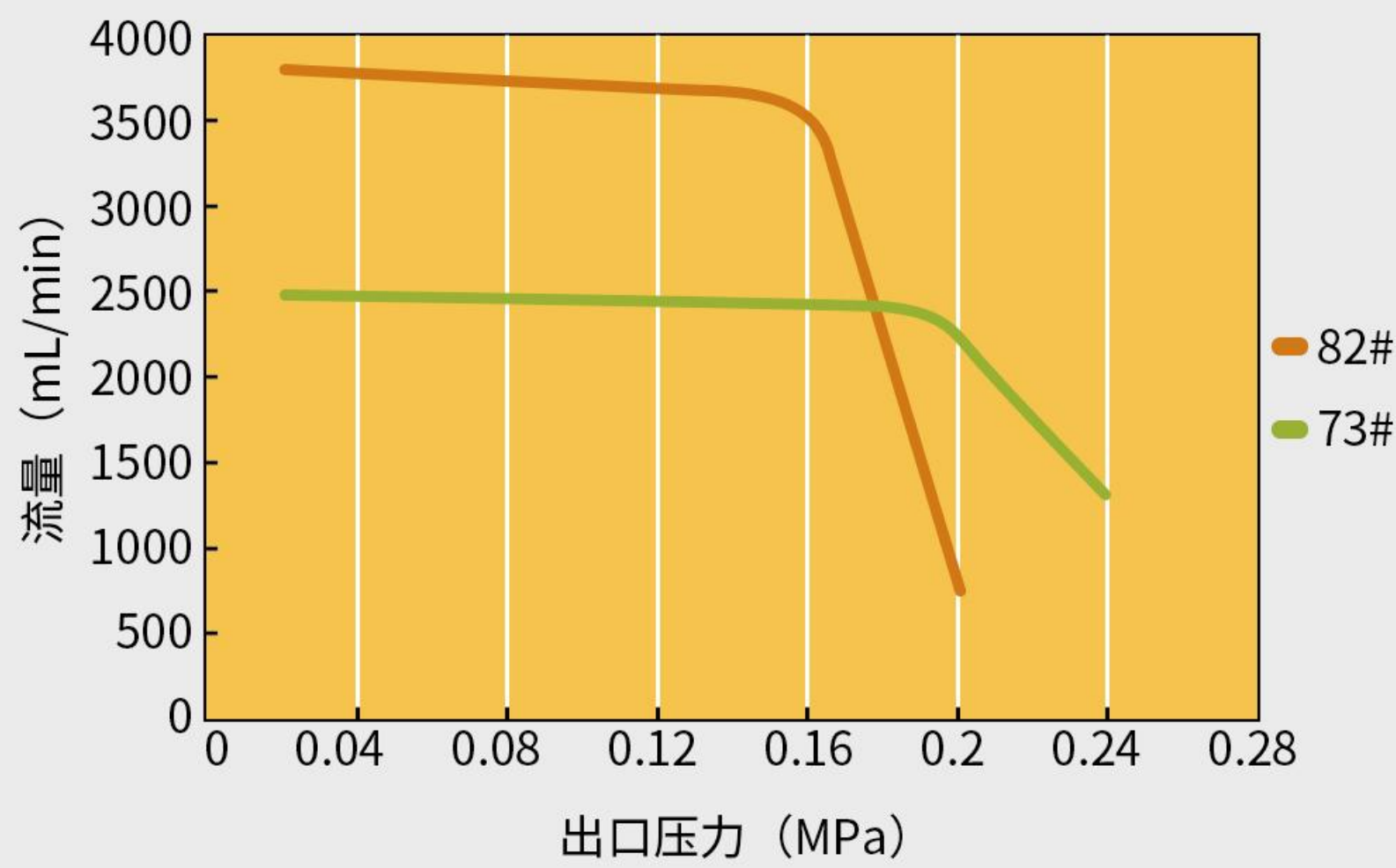
DY35泵头压力/流量曲线图 (100rpm)
