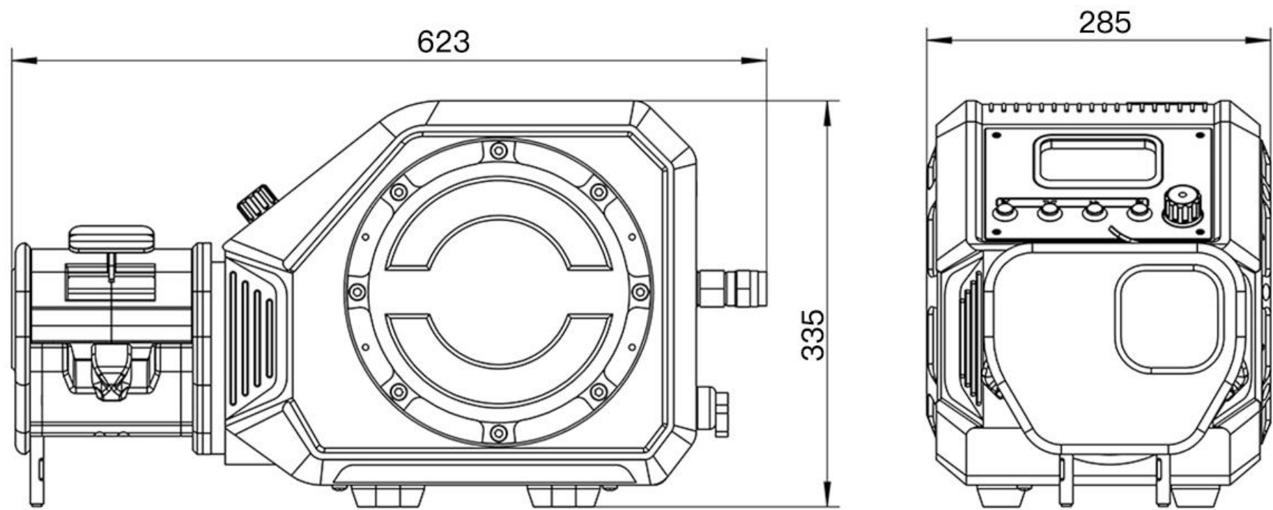
尺寸图 (单位:mm)
