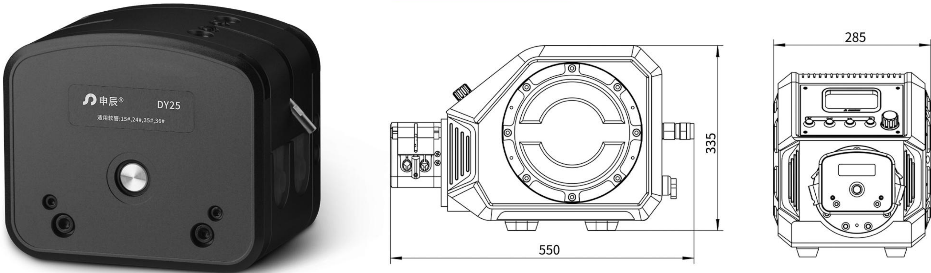
尺寸图 (单位:mm)
