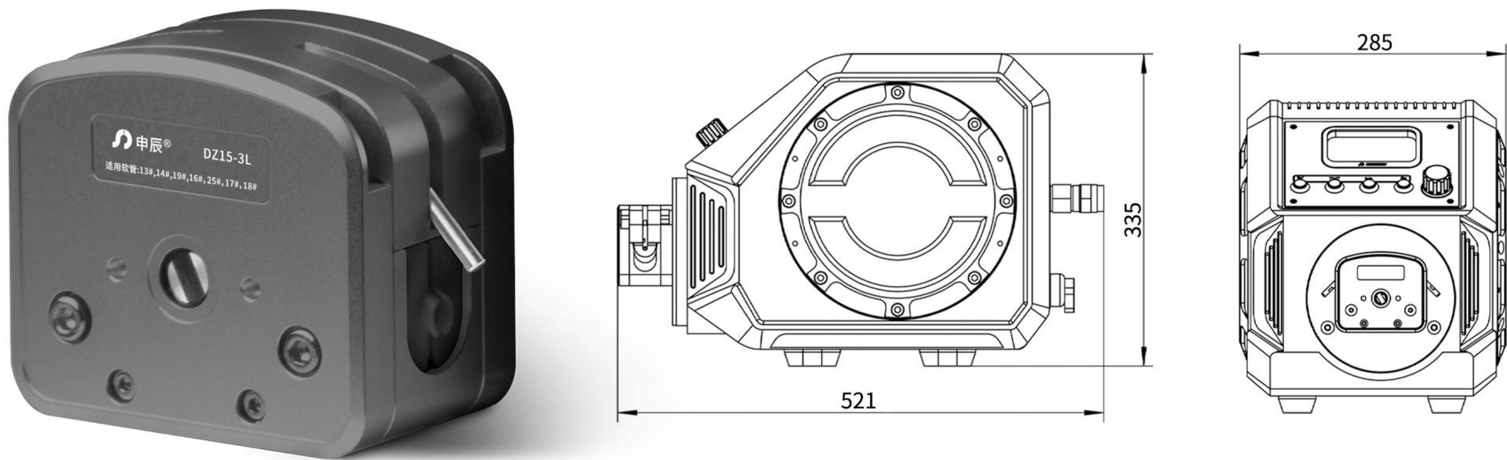
尺寸图 (单位:mm)
