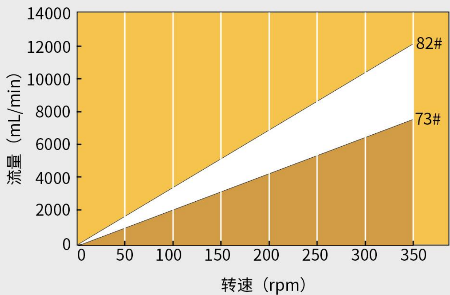
DY35泵头流量范围 (0.1-350rpm)
