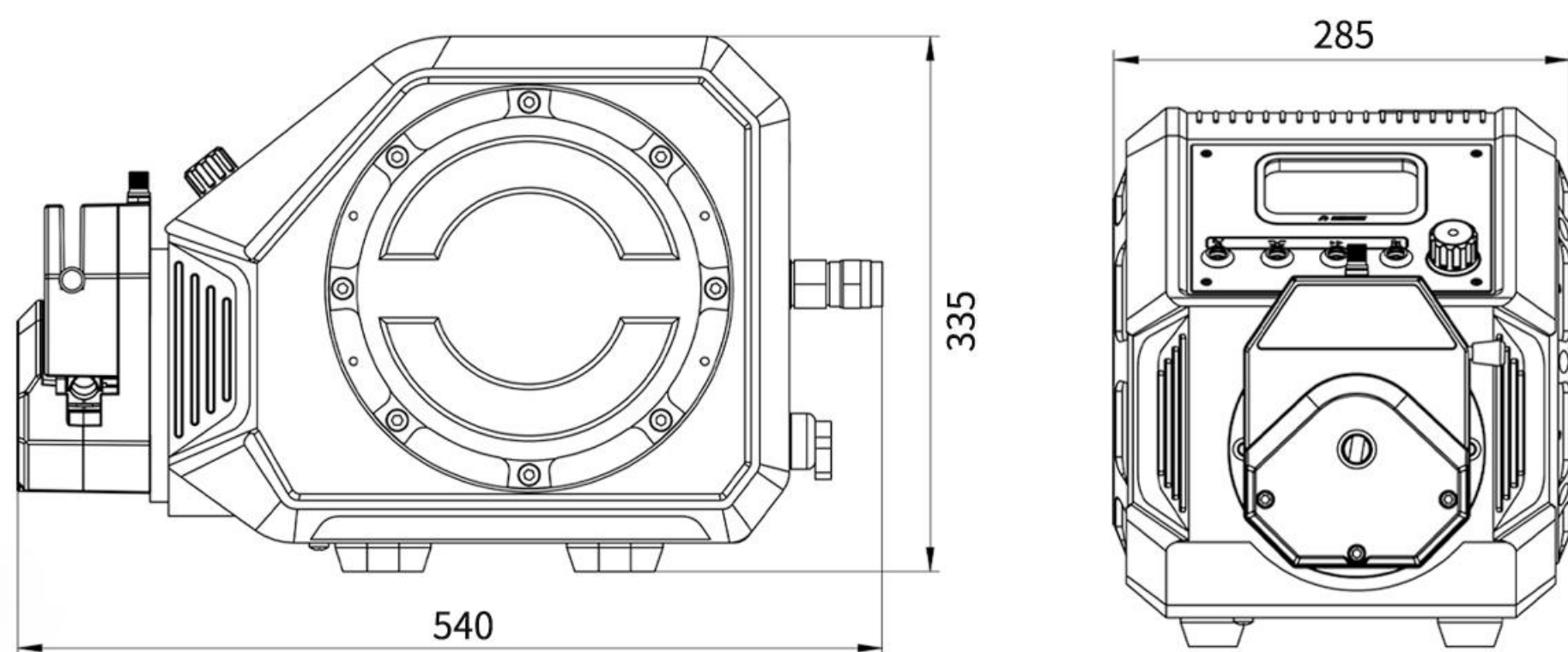
尺寸图 (单位:mm)
