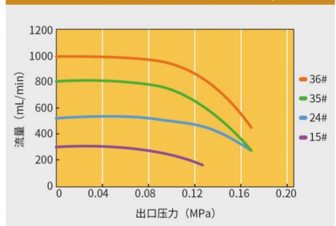
DZ25-6L泵头压力/流量曲线图 (100rpm)
