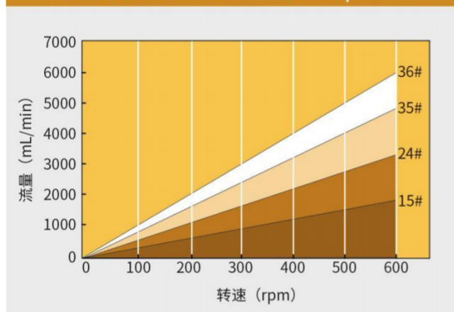
DZ25-6L泵头流量范围 (0.1-600rpm)
