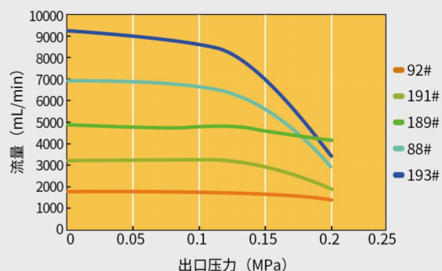
DZ45泵头压力/流量曲线图 (100rpm)
