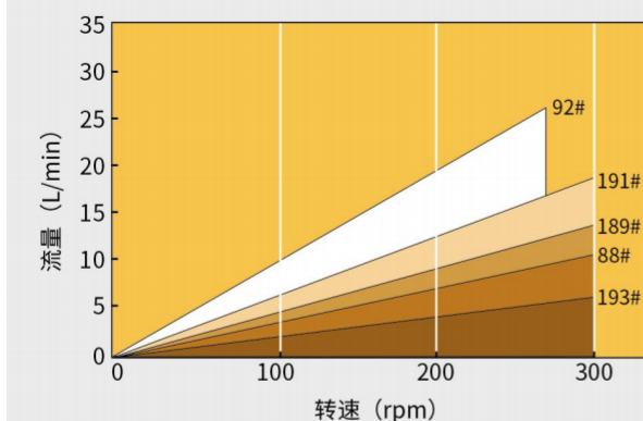
DZ45泵头流量范围 (0.1-300rpm)
