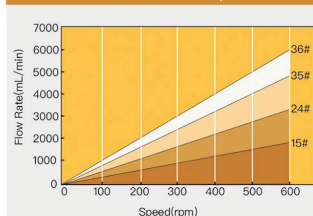
Flow Rate(0.1-600rpm)
