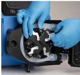
3. 旋转滚轮总成，将滚轮通过板杆扳到工作位置。
