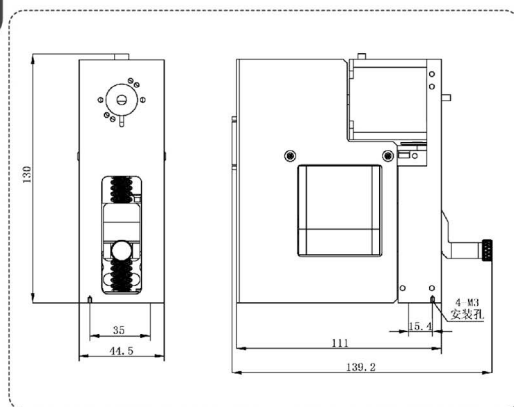
尺寸图(mm)
