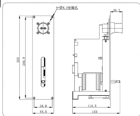
尺寸图(mm)
