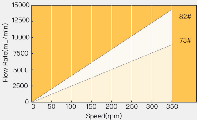
DY Pump Head Filling Volume Reference Parameter
