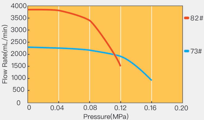
DY Pump Head Filling Volume Reference Parameter
