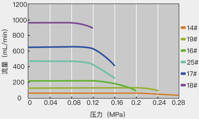
DY15泵头压力/流量曲线图 (100rpm)
