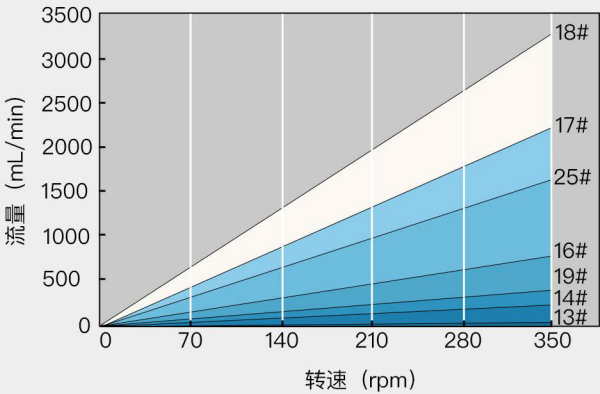
DY15泵头流量范围 (0.1–350rpm)
