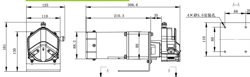
外形尺寸图 (单位: mm)
