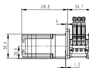
外形尺寸图 (单位: mm)
