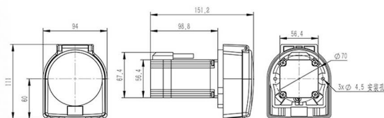
尺寸图 (单位:mm)
