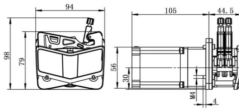
外形尺寸图 (单位: mm)
