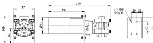
外形尺寸图 (单位: mm)
