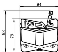
外形尺寸图 (单位: mm)
