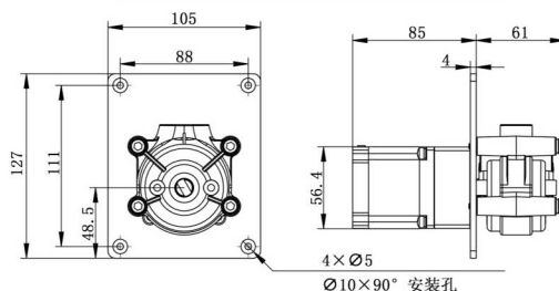
外形尺寸图 (单位: mm)
