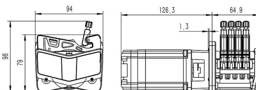
外形尺寸图 (单位: mm)
