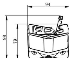
外形尺寸图 (单位: mm)
