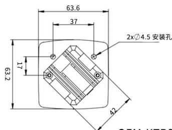
OEM-KTB016尺寸图
