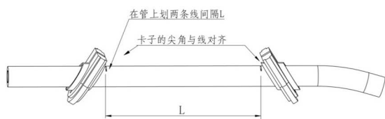
尺寸图
