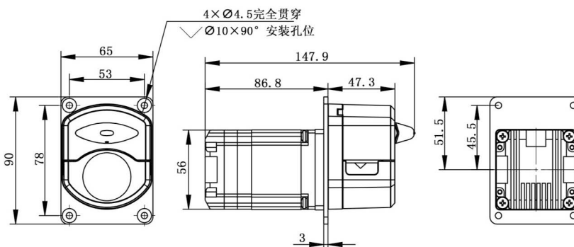
外形尺寸图 (单位: mm)
